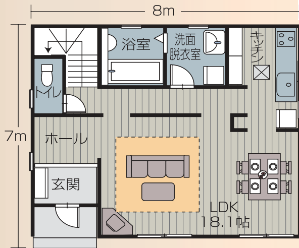
《1F平面図》
