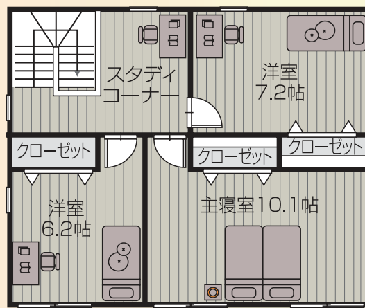
《2F平面図》
